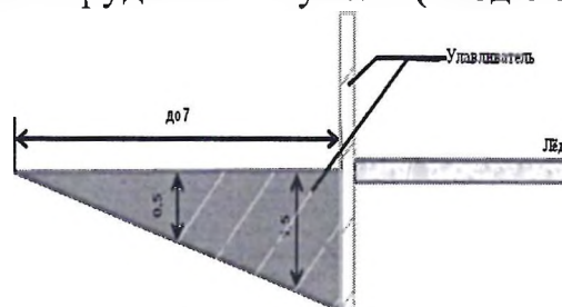
Схема оборудования купели (вход с берега)
